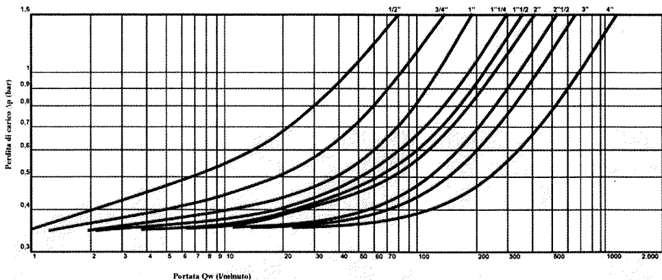
Graf průtoku a odporových ztrát - Graf prietoku a odporových strát DIAGRAMMA DI PORTATA E PERDITA DI CARICO - DISCHARGE AND HEADLOSS DIAGRAM
